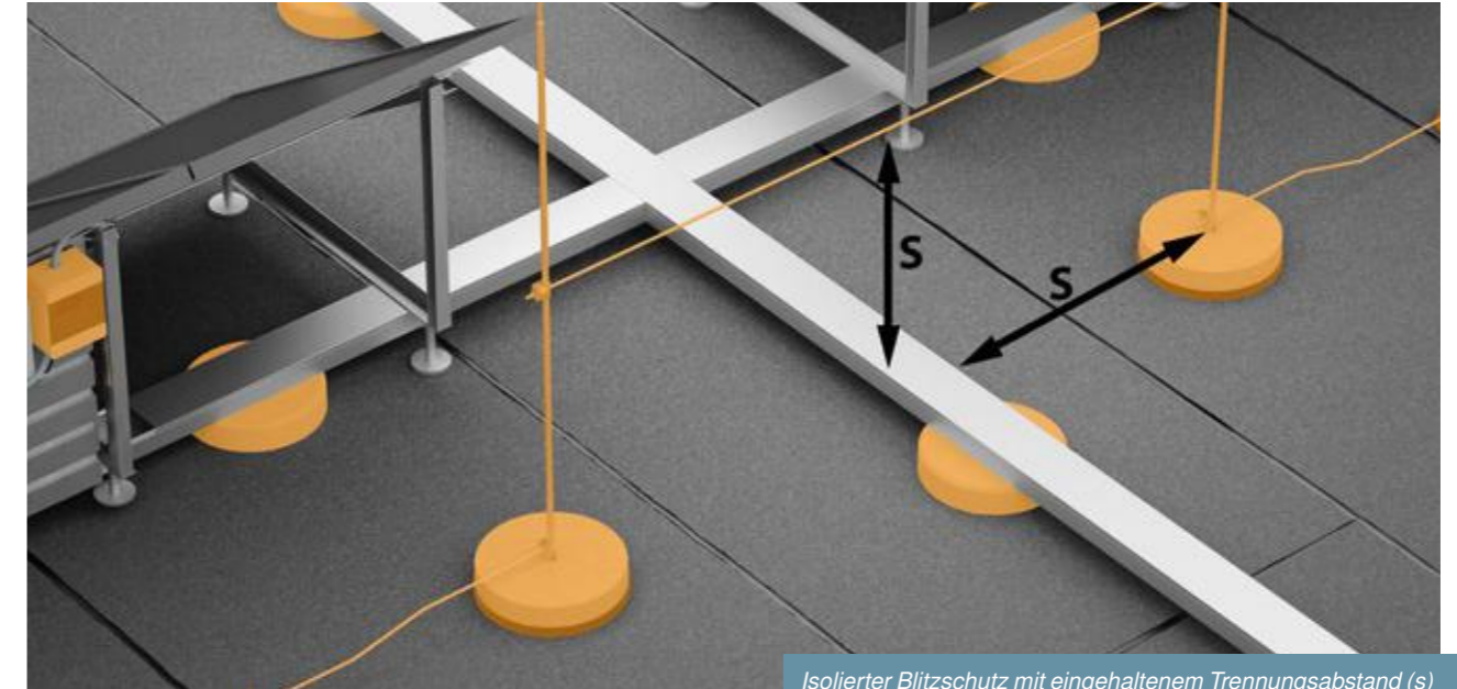
Isolierter Blitzschutz mit eingehaltenem Trennungsabstand (s)
