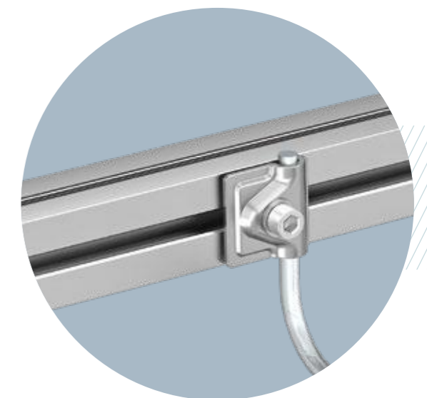
Blitzschutzpotentialausgleich an PV-Montagesystem
