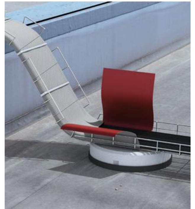
Brandschutzbandage zur Verhinderung der Brandübertragung
