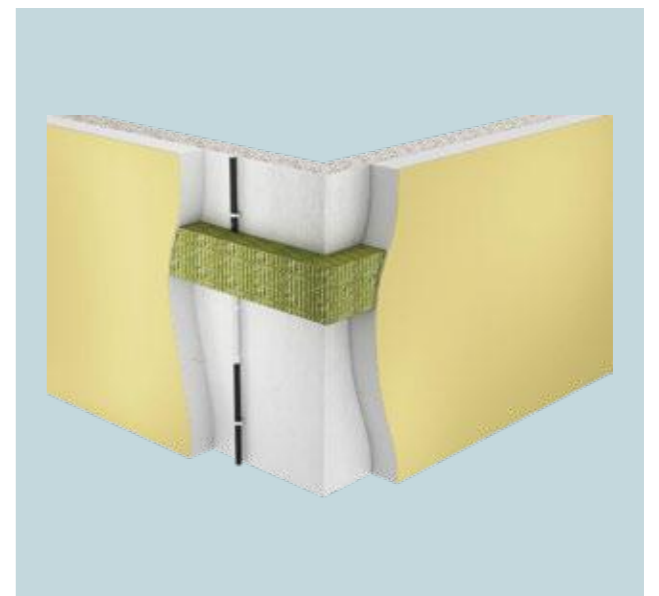
Brandschutzbandage zur Verhinderung der Brandübertragung über isCon® im WDVS
