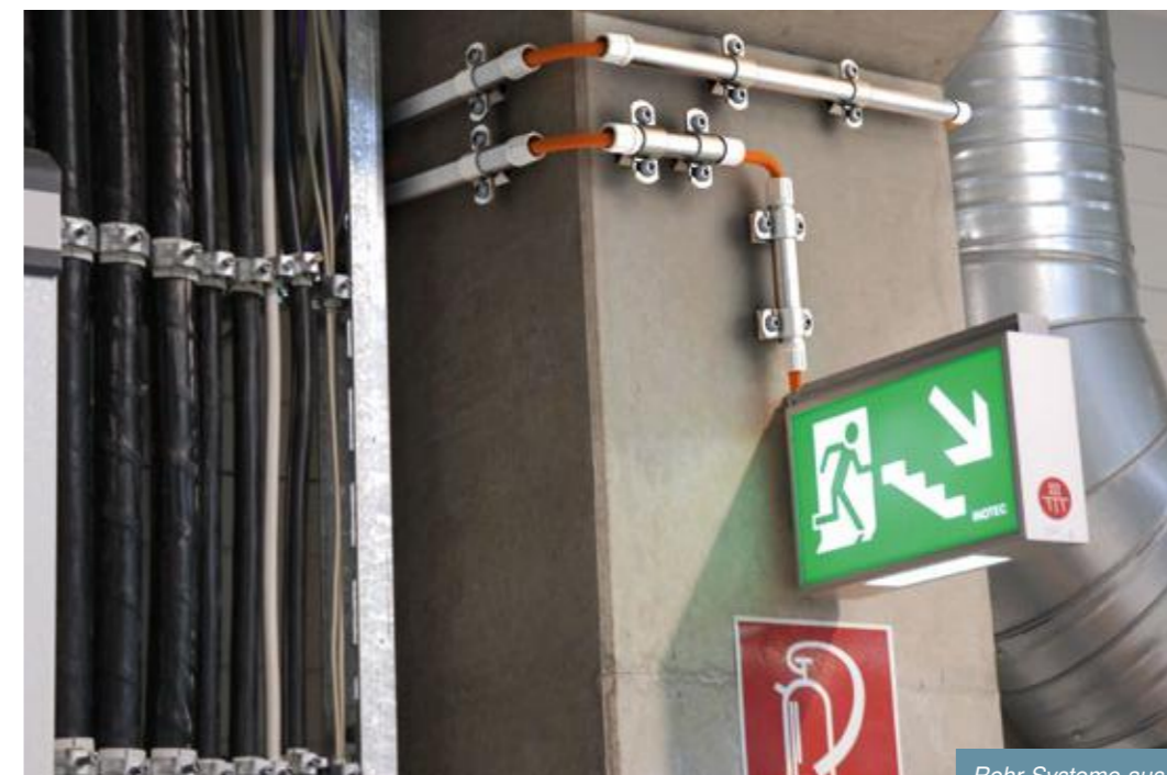
Rohr-Systeme aus Metall: erste Wahl für den Schutz unter harten Bedingungen
