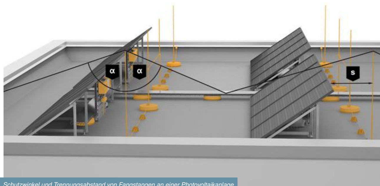
Schutzwinkel und Trennungsabstand von Fangstangen an einer Photovoltaikanlage
